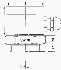
Typ / Type RVA-VVA-A2-AA(PO) = Rohr geschweißt Pipe welded
