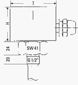
Typ / Type RVA-VVA-A 1/2-AA(PO) = Rohr geschweißt Pipe welded
